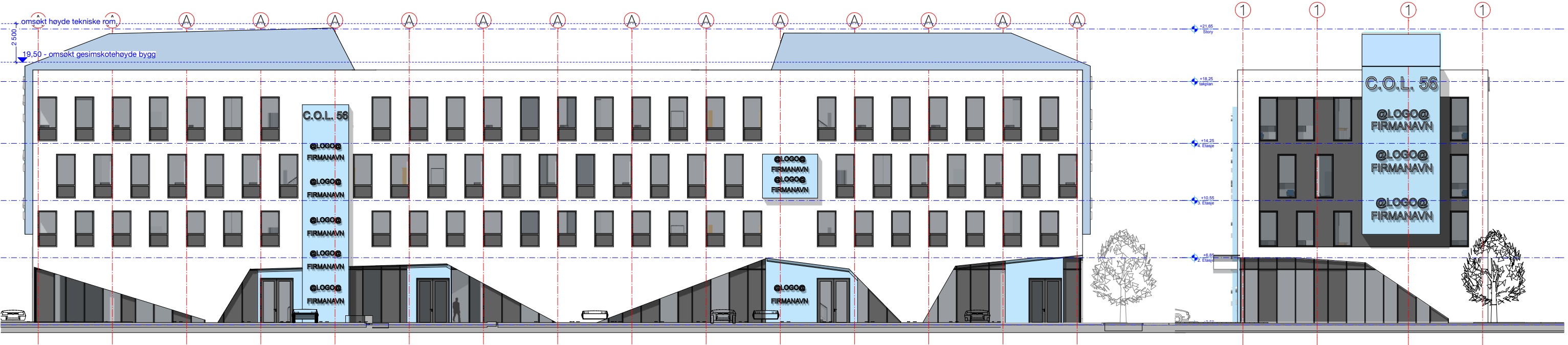
fasade øst
